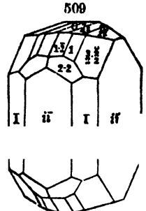
Mt. Doré.
